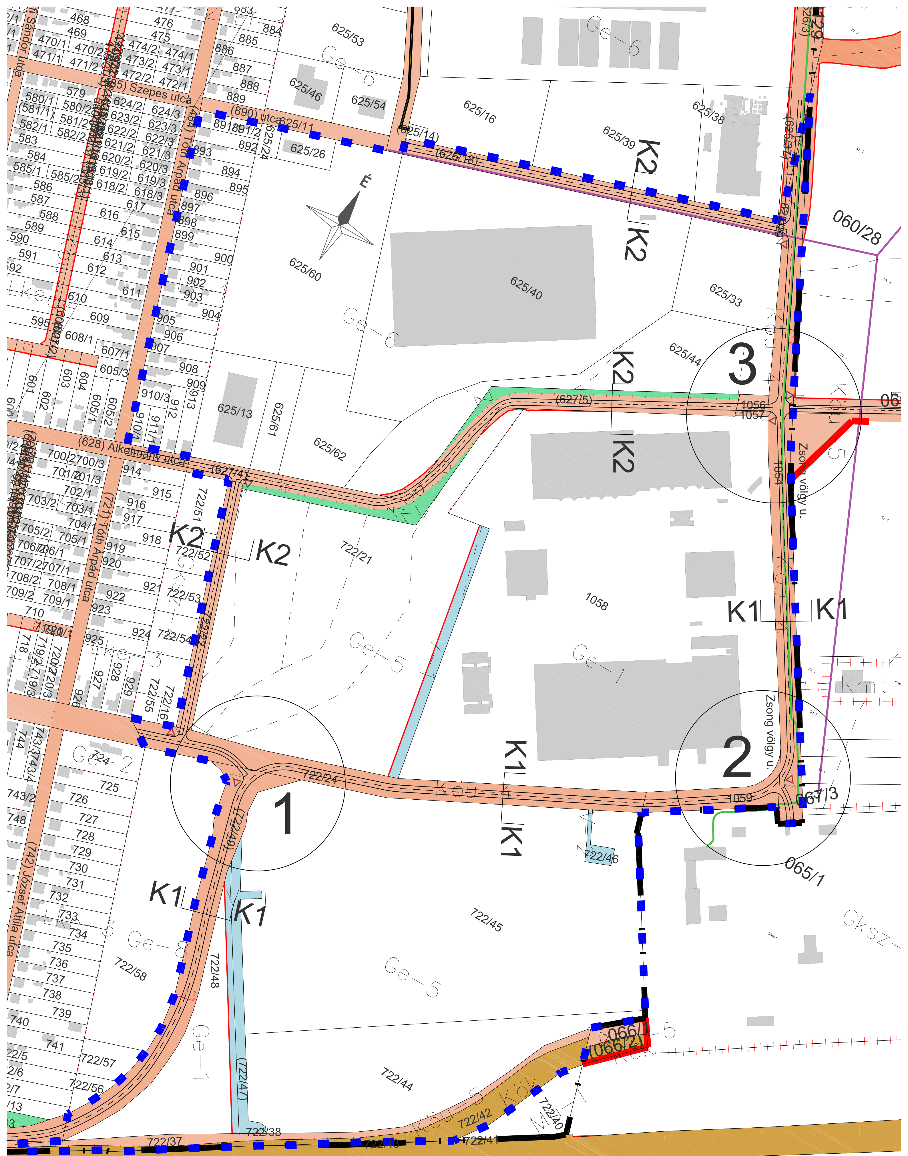
KÖZLEKEDÉS ÁTNÉZETI VÁZLAT M=1:2000
