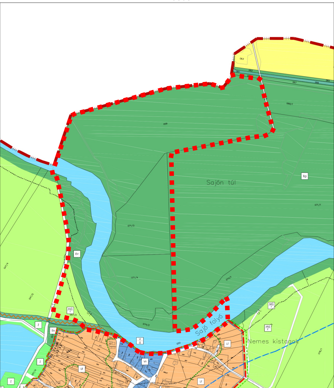
Hatályos szerkezeti terv részlet M = 1 : 8000
