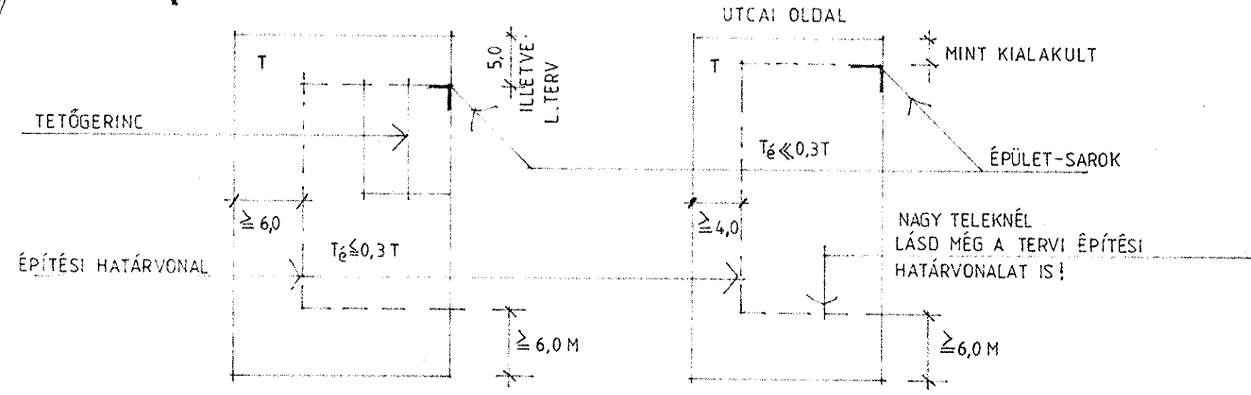
RAJZI MAGYARÁZAT A HÉSZ 6.§-HOZ /ÉPÍTÉSI HELY ÉRTELMEZÉSE/
