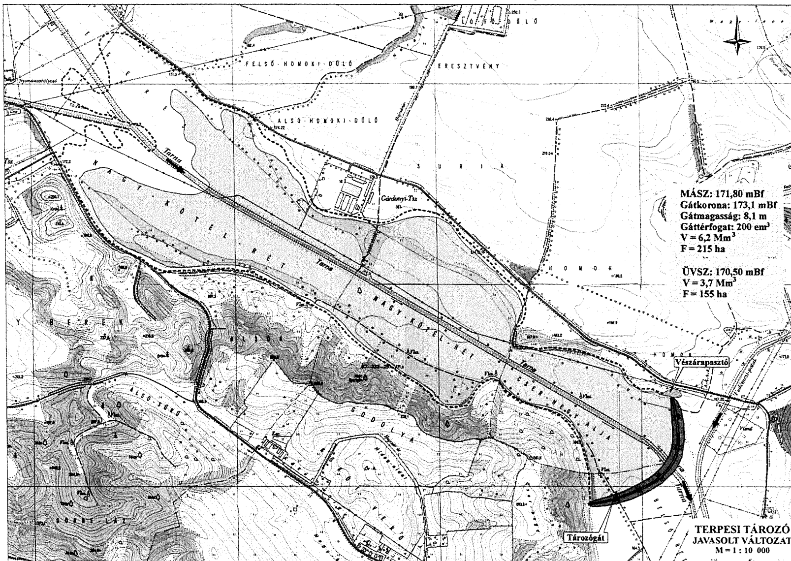
3. ábra A tervezett fejlesztések helyszínrajza
