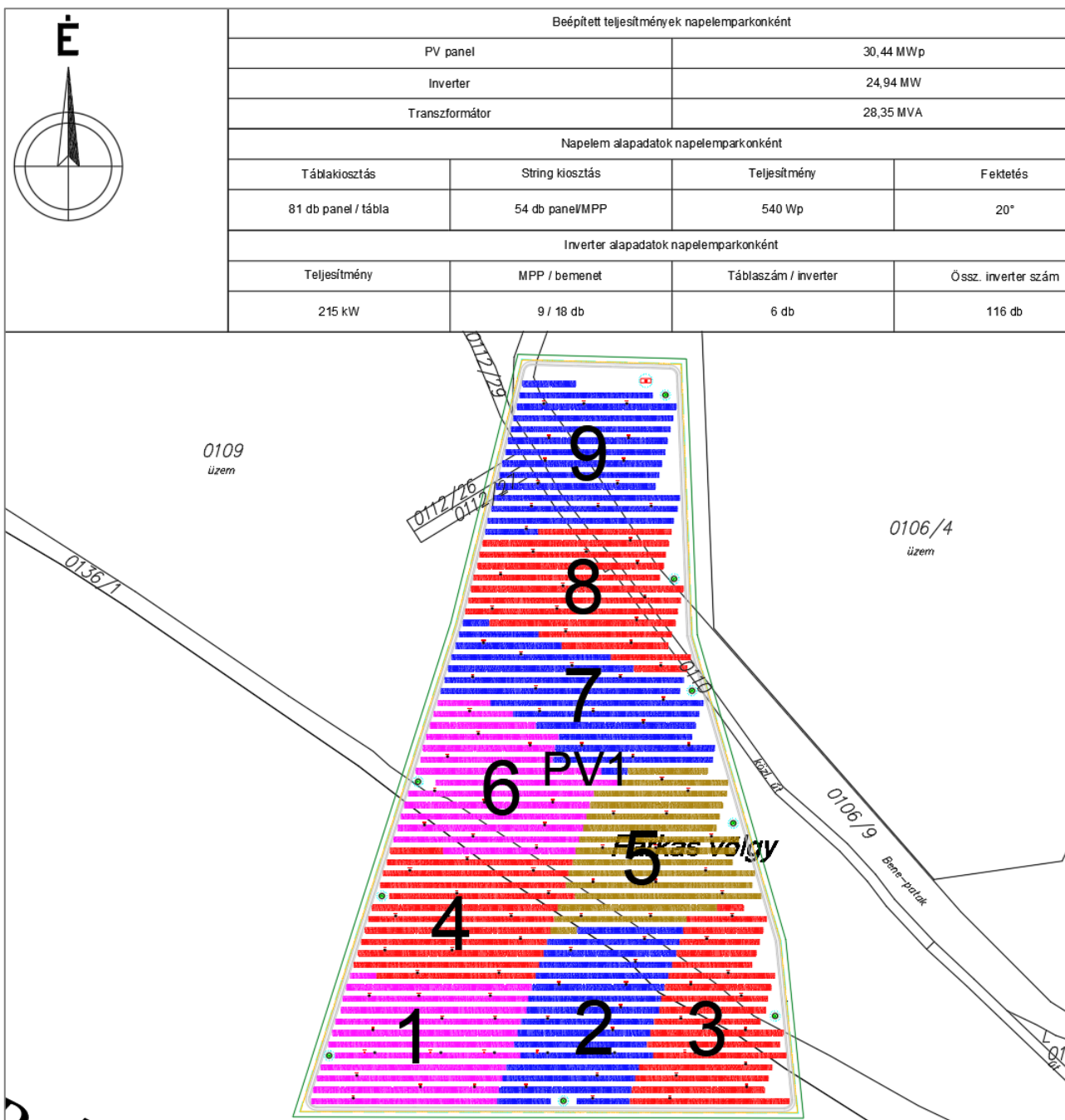
4-1. ábra A naperőmű telepítési elrendezése 20°-os kiosztás esetén
