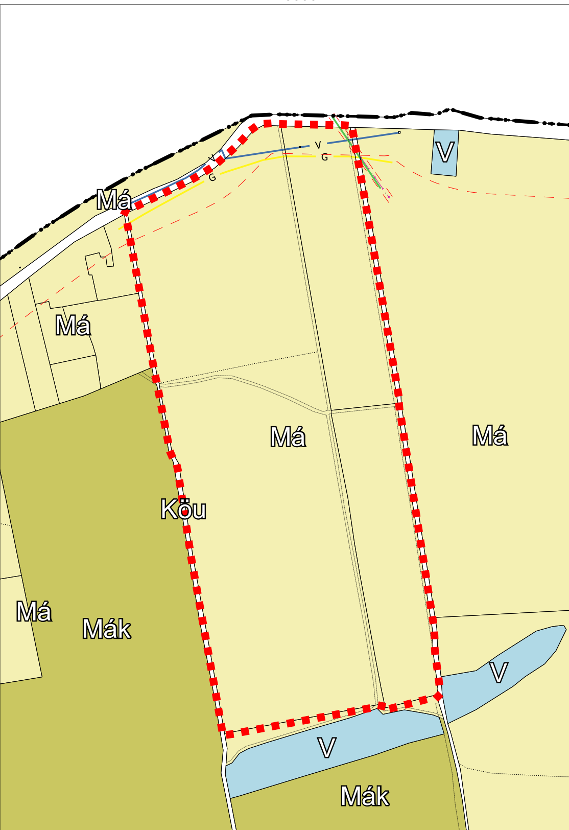
Hatályos szerkezeti terv részlet M 1:6000
