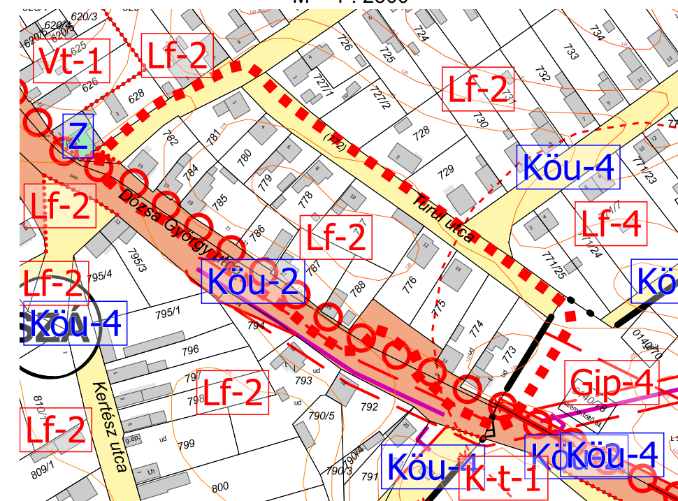
Hatályos szabályozási terv részlet M = 1 : 2500
